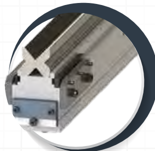
Europäischer Typ Unterwerkzeug (4V Matrizze)
