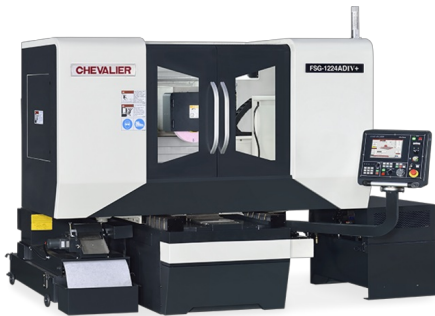
FSG-1224ADIV+ mit Volleinhausung
