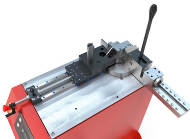
Mit Biegevorrichtung AB-PF zum Winkelbiegen
