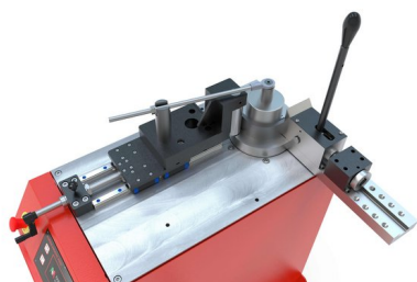
Mit Biegevorrichtung AB-CF zum Rundbiegen
