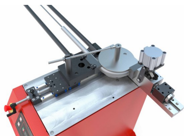
Mit Biegevorrichtung AB-CTA zum Rohrbiegen mit Dorn mit pneumatischer Spannvorrichtung
