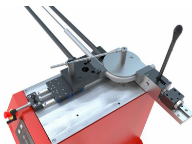
Mit Biegevorrichtung AB-CTA zum Rohrbiegen mit Dorn mit manueller Spannvorrichtung
