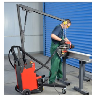
Entlastungs- / Hebe-Set
