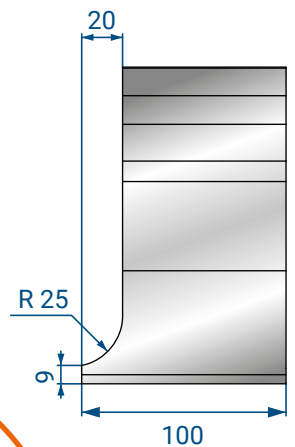
HORNSTÜCK
