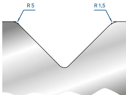
RADIENÄNDERUNG
