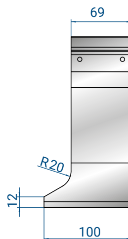
HORNSTÜCK
