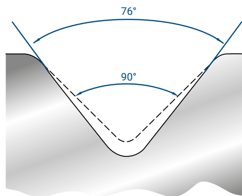
WINKELÄNDERUNG
