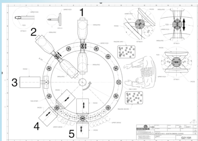
Smerigliatrice a giostra a 9 teste con nastro abrasivo e spazzole per la pulitura di pezzi di 40 mm
