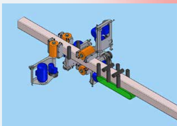
Spazzolatrice a quattro teste per la pulitura di tubi quadri con guida tramite rulli
