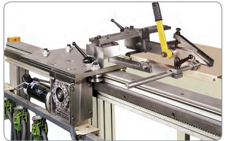
Vorschubeinheit PAX
