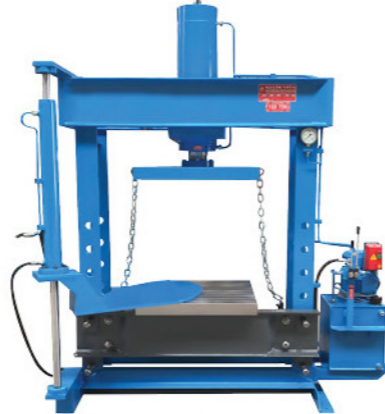
Forklift Lastiği Sökme Presi Forklift Tire Press
